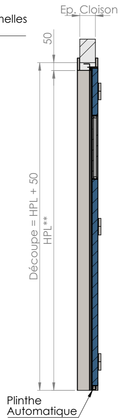
COUPE B-B
